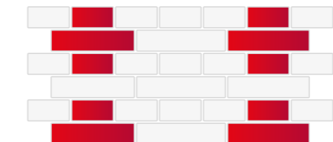
WIĄZANIE KRZYŻOWE TYP 1
