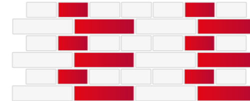
WIĄZANIE BLOKOWE
