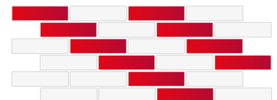
WIĄZANIE WOZÓWKOWE PRZESUNIĘCIE O 1/4 CEGŁY
