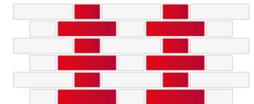
WIĄZANIE WOZÓWKOWE PRZESUNIĘCIE O 1/2 CEGŁY
